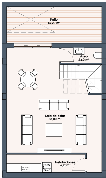
Planta Sótano
