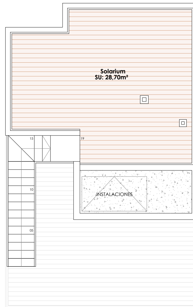
PLANTA CUBIERTA
