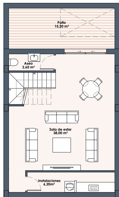
Planta Sótano
