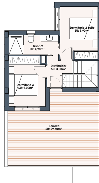
Planta Primera
