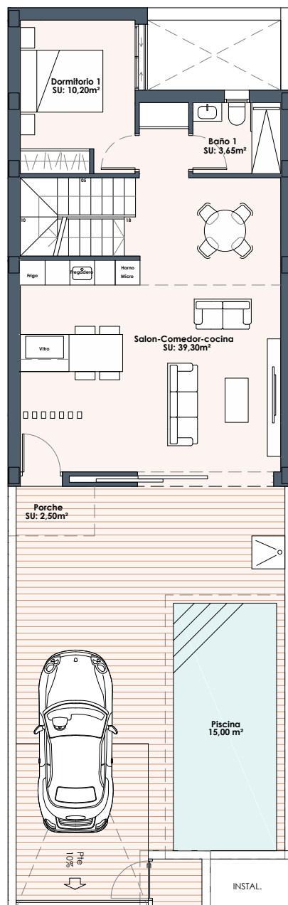
Planta Baja
