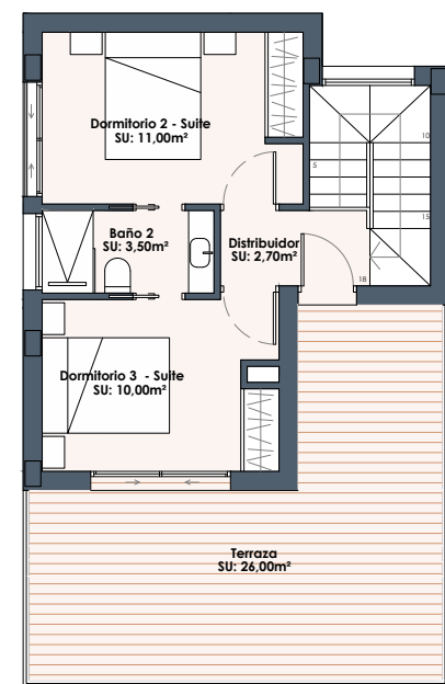
Planta Primera
