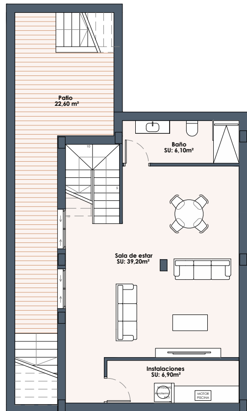
Planta Sótano
