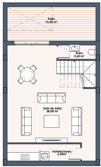
Planta Sótano
