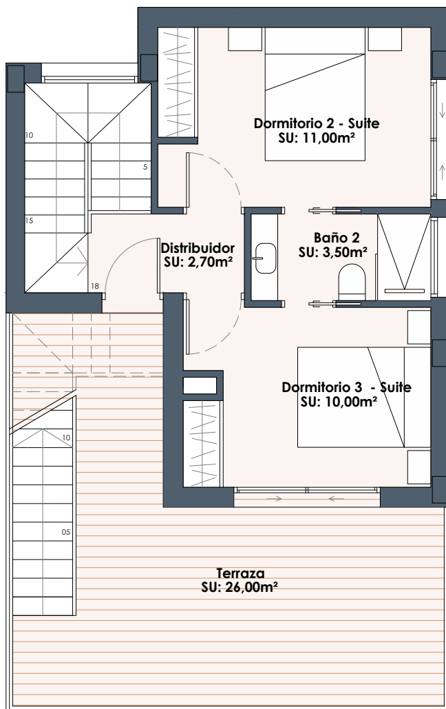
PLANTA PRIMERA
