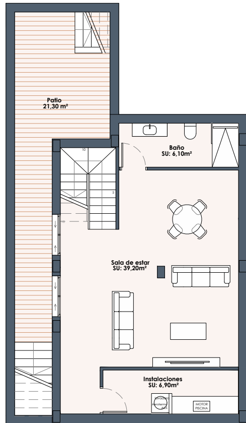
Planta Sótano
