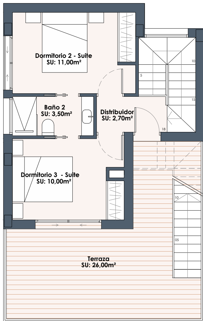
PLANTA PRIMERA
