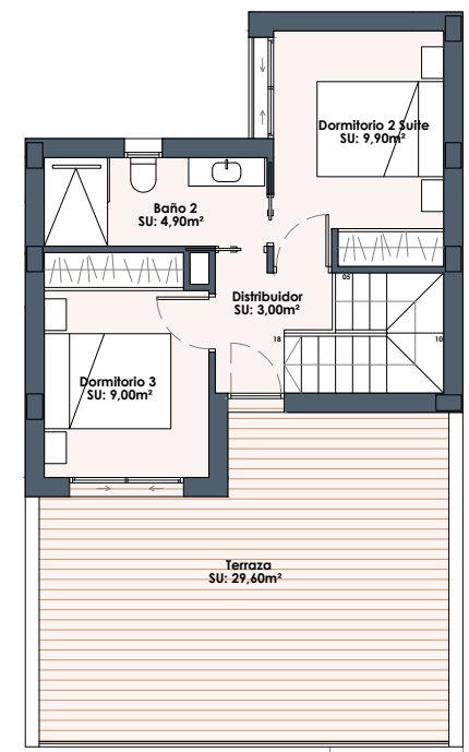
Planta Primera
