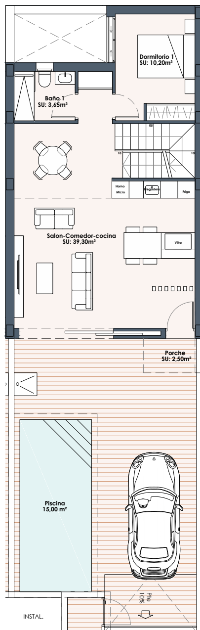
Planta Baja
