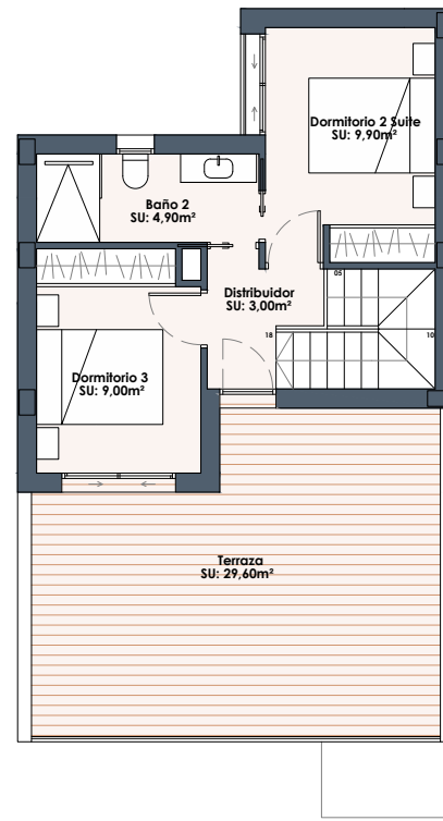
Planta Primera
