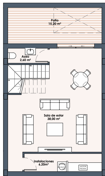
Planta Sótano
