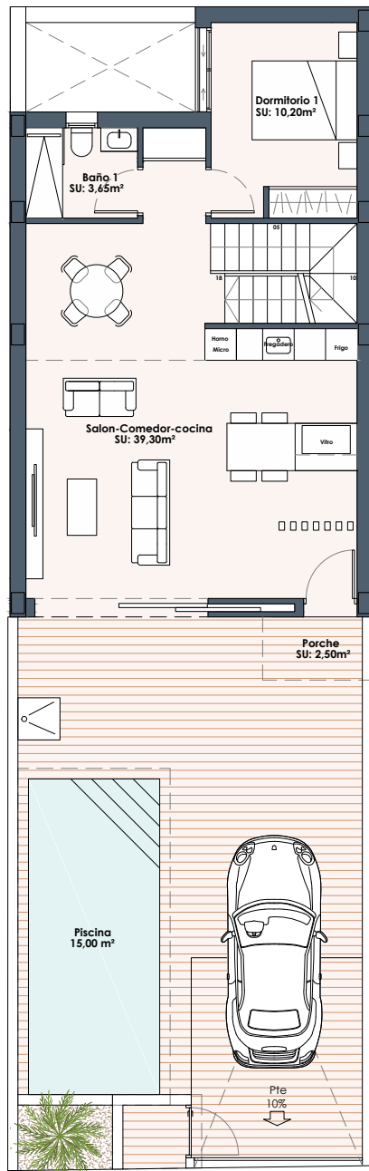
Planta Baja
