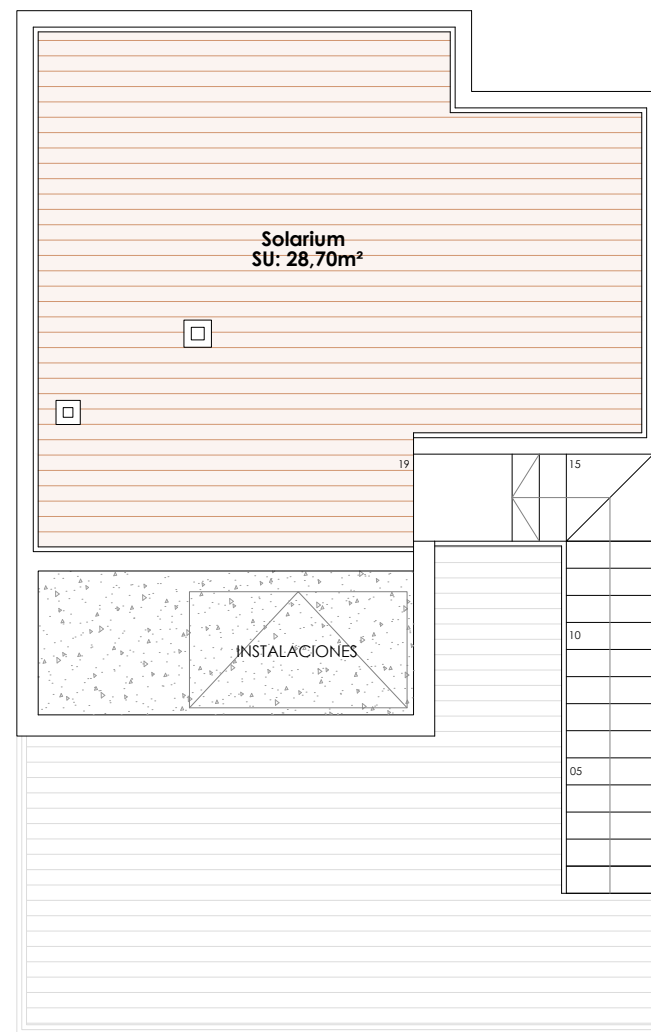
PLANTA CUBIERTA
