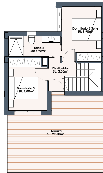
Planta Primera
